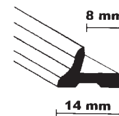
vnitřní rohový profil
