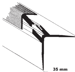
typ B, výška krytiny 9 - 16 mm základní + vrchní profil
