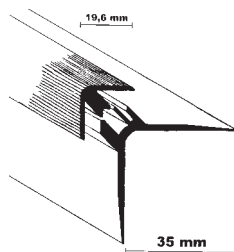
typ A, výška krytiny 5 - 9 mm základní + vrchní profil
